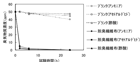
図3 脱臭繊維布の試験結果
