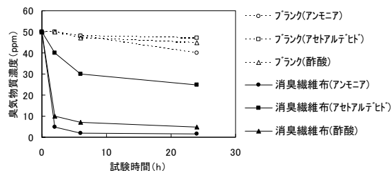
図2 消臭繊維布の試験結果
