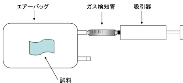
図1 試験の概略図
