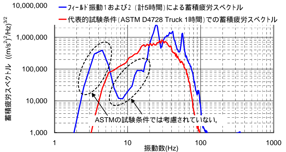
図3 輸送シナリオ(フィールド振動1および2)と代表的試験条件(ASTM)の比較
