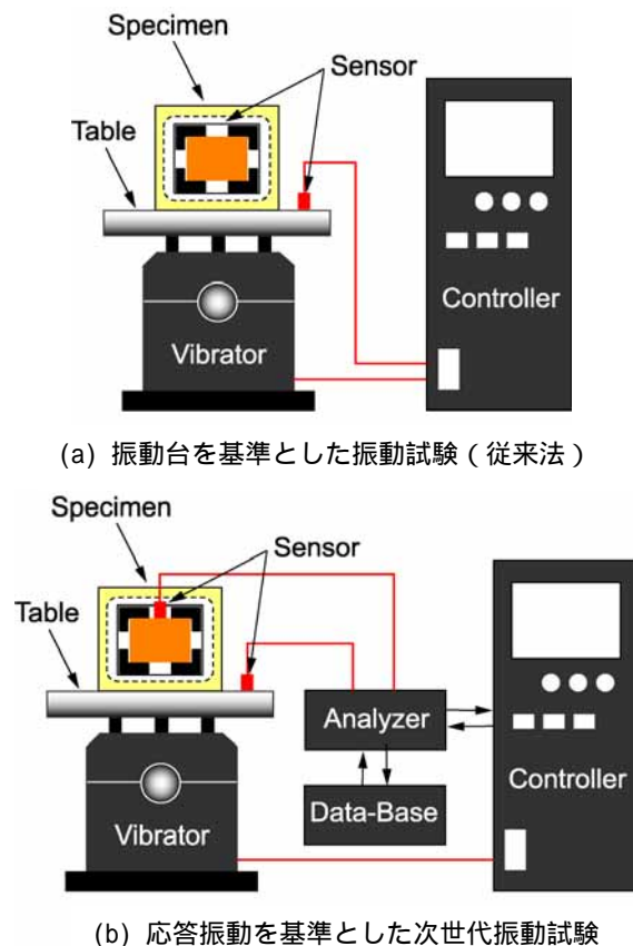
図1 従来型振動試験と次世代振動試験
