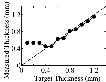
図5 壁厚さの実測値と設計値の関係
