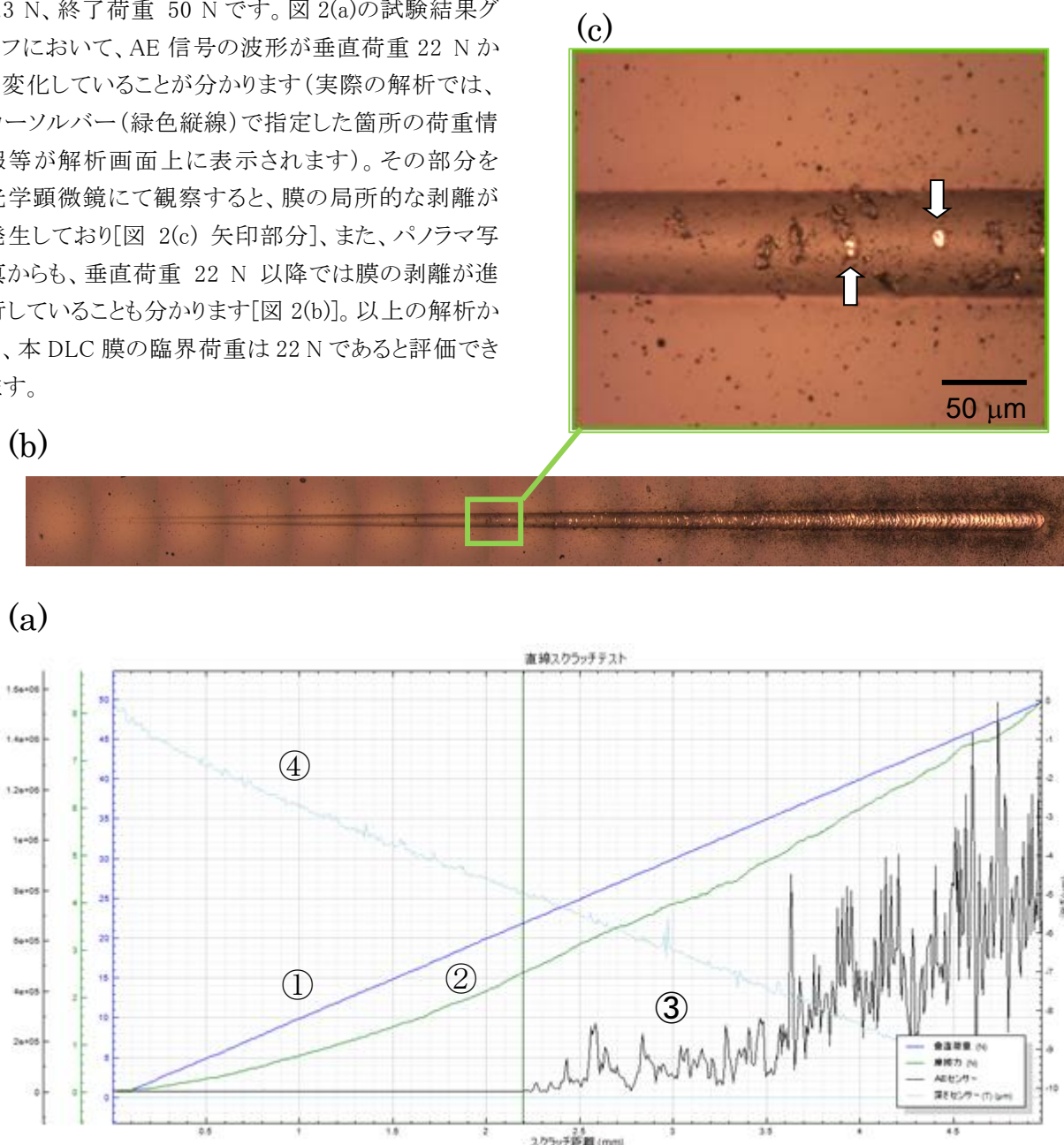
① 垂直荷重 (N), ② 摩擦力(N), ③ AE 信号, ④ 深さ(μm)
