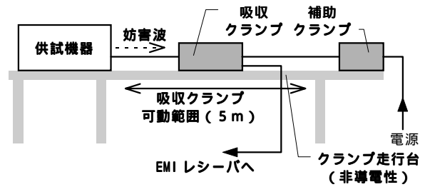
図6 吸収クランプによる妨害電力の測定
