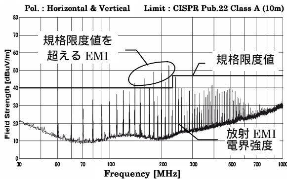
図5 放射 EMI 測定の速定例
