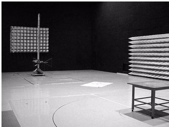
図4 電波暗室の内部
