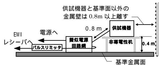
図 2 伝導 EMI 測定の模式図
