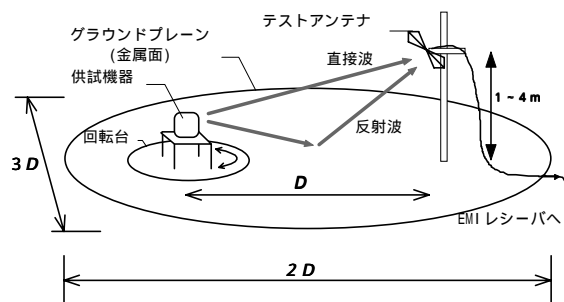
図 3 放射 EMI 測定の模式図(オープンサイト)
