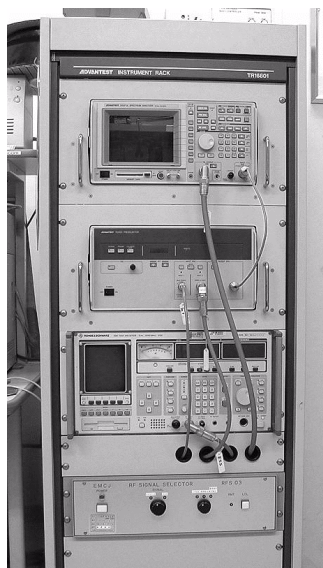
図 1 EMI 測定システム
