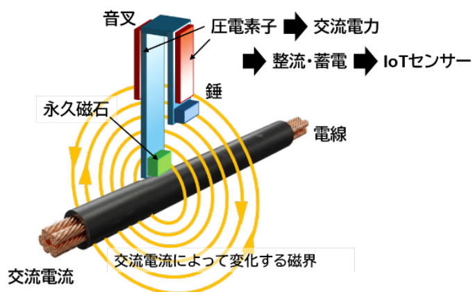
図1 発電の原理
