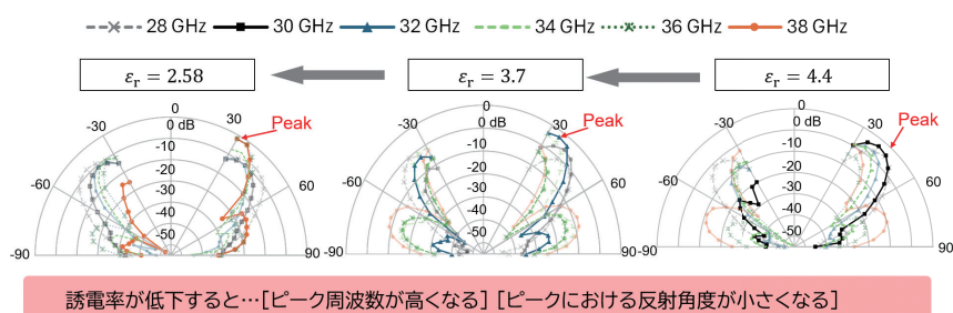
基板誘電率によるメタサーフェス反射特性の変化（測定結果）
