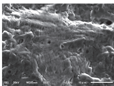
破面画像
