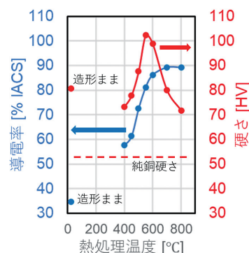
熱処理後の造形体の 導電率と硬さ
