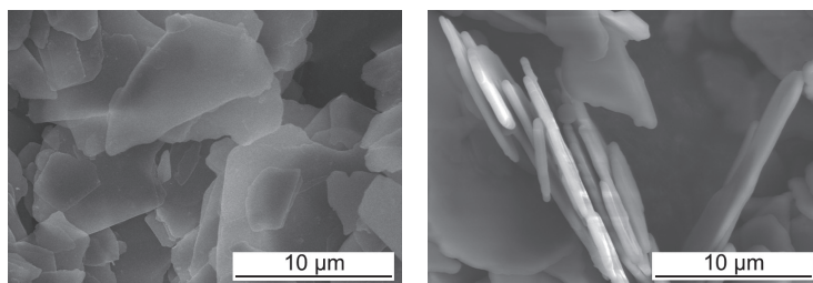
マイカ粒子
