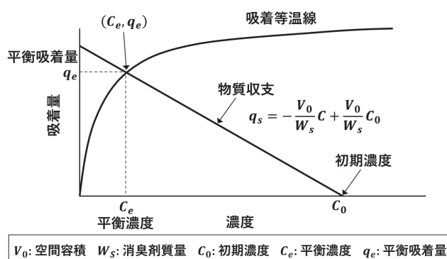
吸着等温線と物質収支の関係
