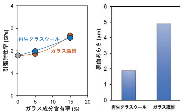
ガラス添加材料の引張弾性率 ガラス成分5%品の表面あらさ
