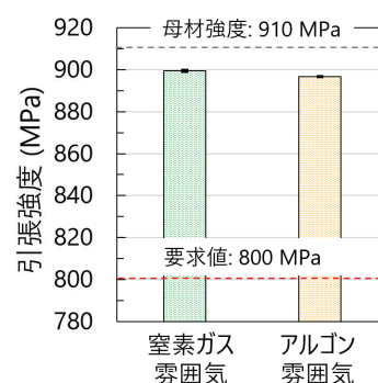
レーザ溶接試験体の強度
