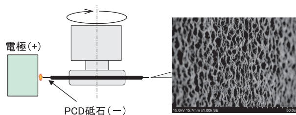
放電加工による微小切れ刃とチップポケットの形成
