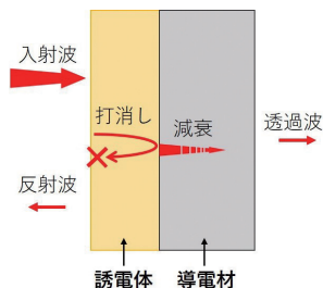
構造模式図
