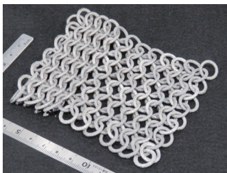
電子ビーム積層造形物 (チタン合金製の継ぎ目のない鎖)
