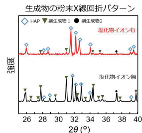
生成物のX線回折パターン
