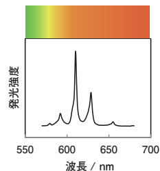
Eu付与ジルコニア結晶集合体の発光スペクトル
