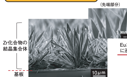
Zr水溶液の電気分解で得られた結晶体
