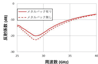
電磁波吸収特性
