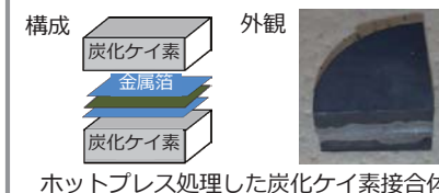
構成 炭化ケイ素 金属箔 炭化ケイ素 外観 ホットプレス処理した炭化ケイ素接合体
