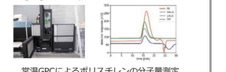
常温GPCによるポリスチレンの分子量測定
