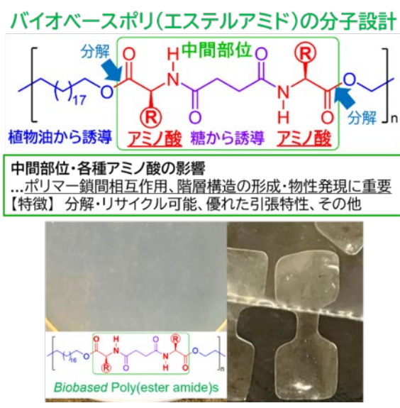
図2 今回開発したバイオベースポリ(エステルアミド)の基本構造。コハク酸(紫色、糖から誘導)、長鎖脂肪酸(植物油より誘導)、アミノ酸を構成単位とし、定量的なケミカルリサイクルが可能(アルコールとのトランスエステル化、青色矢印部位が解離)。下図は調製したバイオベースポリ(エステルアミド)フィルム(溶媒キャスト法)。
