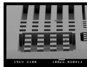
シリコン基板の加工例
