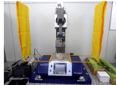
シャルピー衝撃強度測定システム 東洋精機製作所 製
