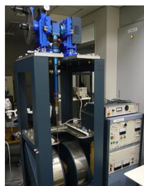
振動試料型磁力計 機器型番：BHV-50 理研電子株式会社 製
