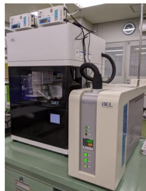
触媒・吸着剤評価装置
