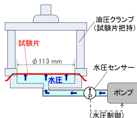
耐水度試験機の主要部模式図
