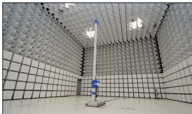
第1電波暗室（10m法）
