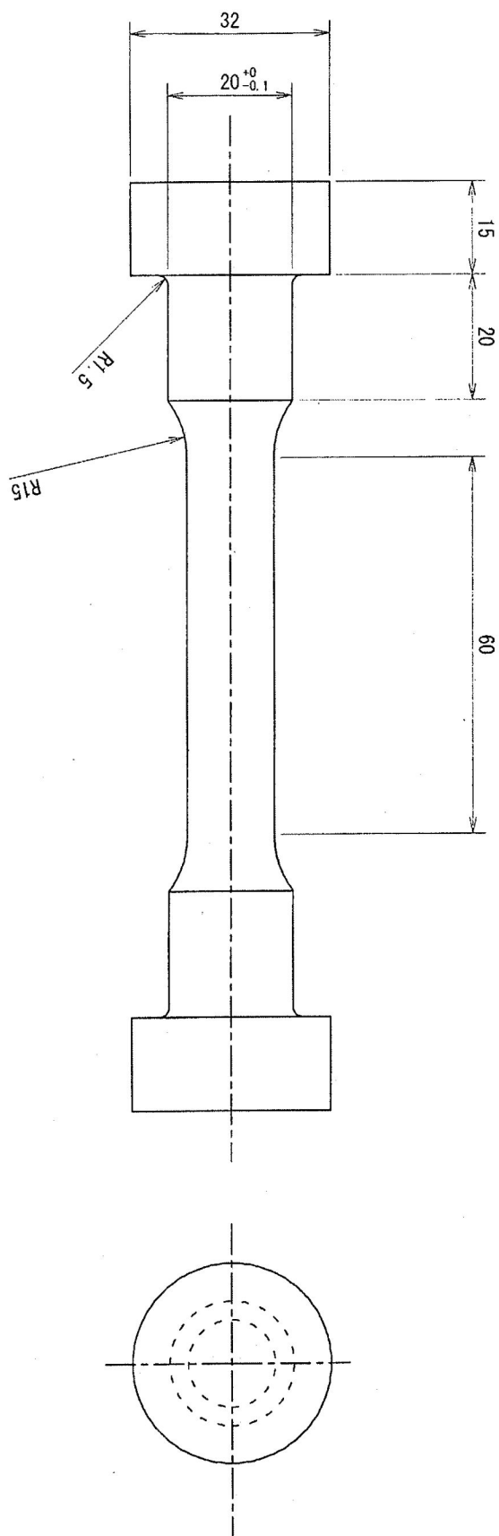
肩付き試験片
